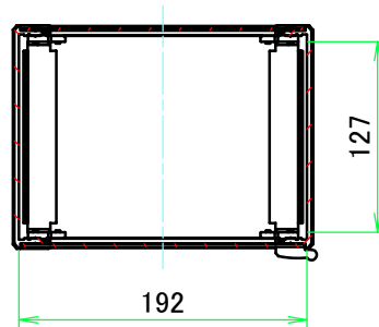
A-A ( 1 : 5.5 )
