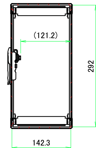
B-B ( 1 : 5.5 )
