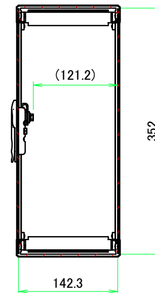
B-B ( 1 : 5.5 )
