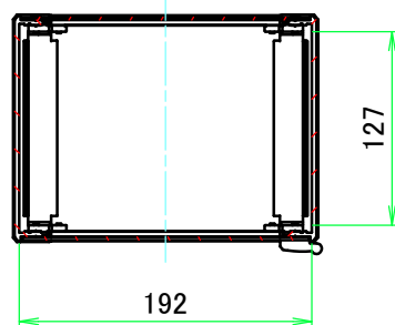
A-A ( 1 : 5.5 )
