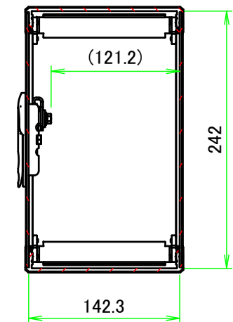
B-B ( 1 : 5 )
