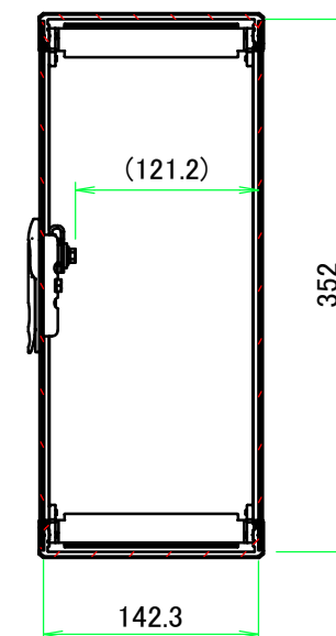
B-B ( 1 : 5.5 )
