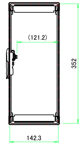
B-B ( 1 : 5.5 )
