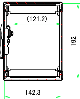
B-B ( 1 : 5 )
