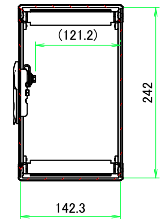
B-B ( 1 : 5.5 )
