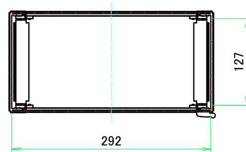
A-A ( 1 : 5.5 )
