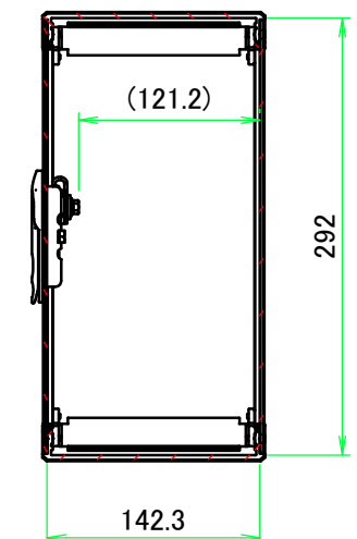
B-B ( 1 : 5.5 )
