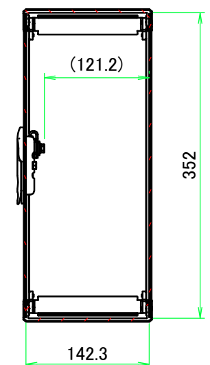
B-B ( 1 : 6 )
