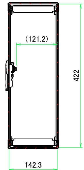
B-B ( 1 : 6.5 )
