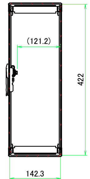
B-B ( 1 : 6.5 )
