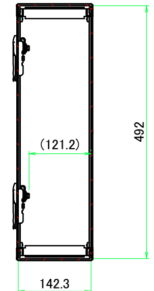
B-B ( 1 : 7.5 )
