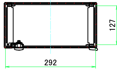
A-A ( 1 : 7.5 )
