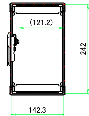
B-B ( 1 : 6 )
