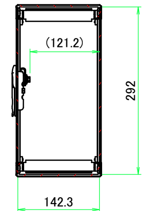
B-B ( 1 : 6.5 )
