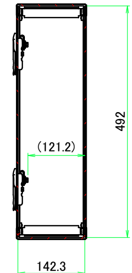
B-B ( 1 : 8 )
