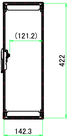
B-B ( 1 : 8 )
