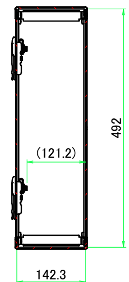
B-B ( 1 : 8 )
