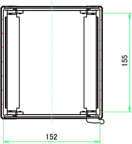
A-A ( 1 : 3.5 )
