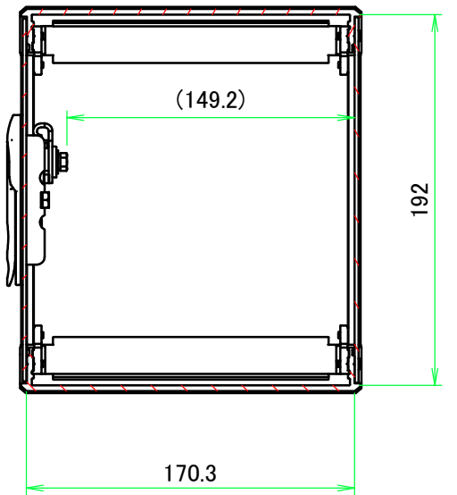
B-B ( 1 : 3.5 )
