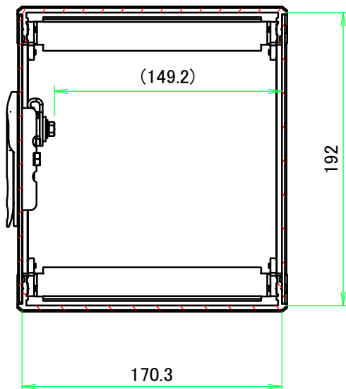
B-B ( 1 : 3.5 )
