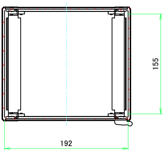
A-A ( 1 : 3.5 )
