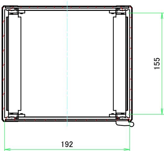
A-A ( 1 : 3.5 )
