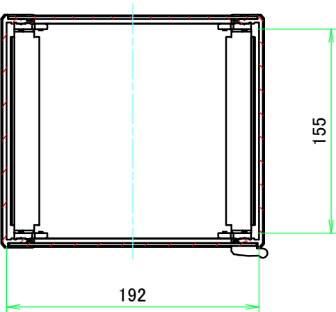
A-A ( 1 : 4 )
