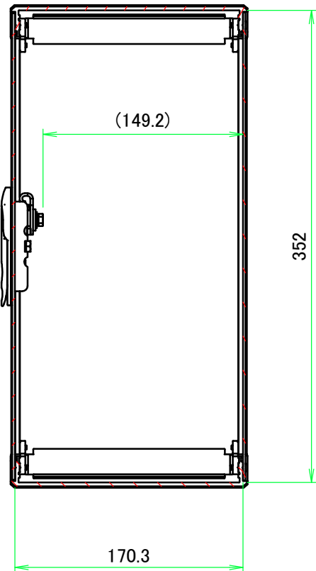
B-B ( 1 : 4 )
