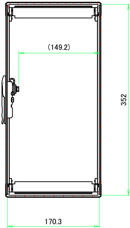
B-B ( 1 : 4 )
