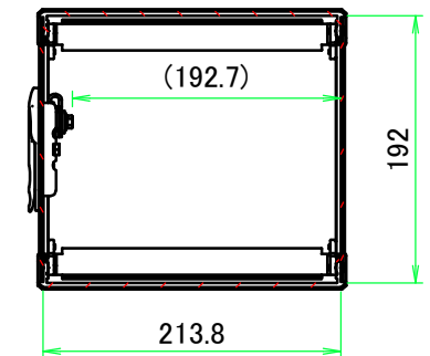
B-B ( 1 : 6 )
