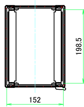
A-A ( 1 : 6 )
