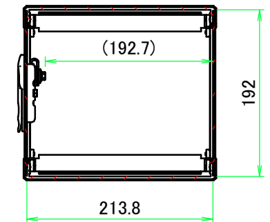
B-B ( 1 : 6 )
