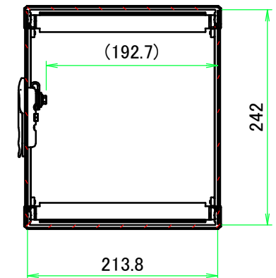
B-B ( 1 : 6 )
