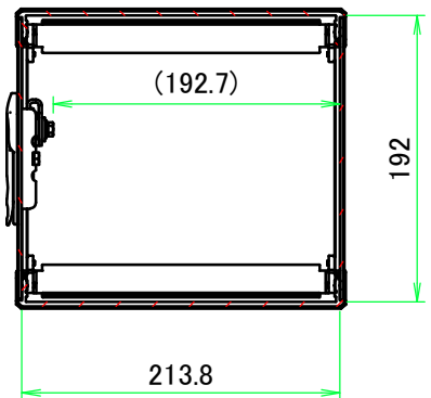
B-B ( 1 : 5.5 )
