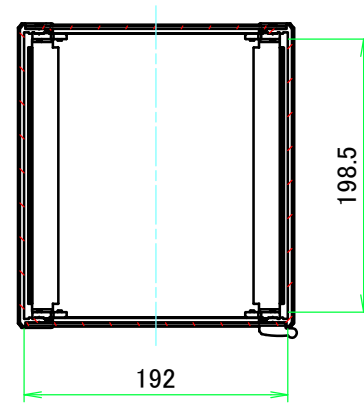
A-A ( 1 : 5.5 )
