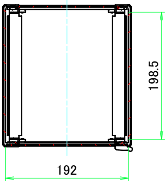
A-A ( 1 : 6 )
