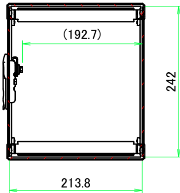
B-B ( 1 : 6 )
