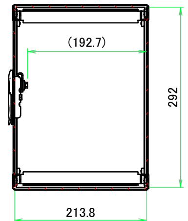
B-B ( 1 : 6 )
