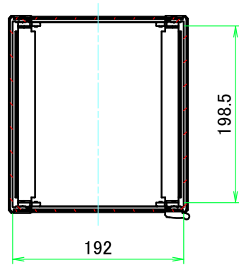
A-A ( 1 : 6 )
