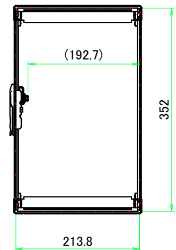
B-B ( 1 : 6.5 )
