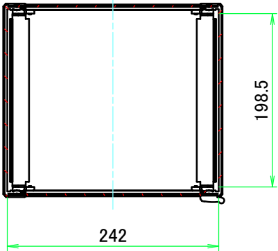
A-A ( 1 : 6 )
