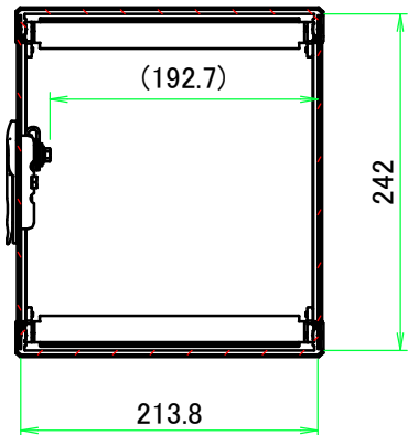
B-B ( 1 : 6 )
