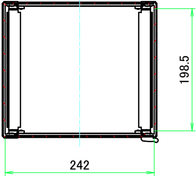
A-A ( 1 : 6 )
