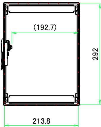
B-B ( 1 : 6.5 )
