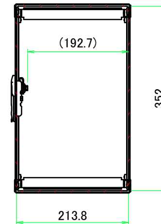
B-B ( 1 : 7 )
