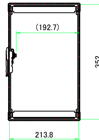
B-B ( 1 : 7 )
