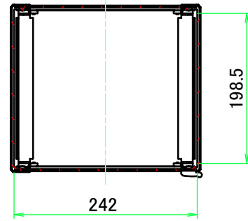
A-A ( 1 : 7 )
