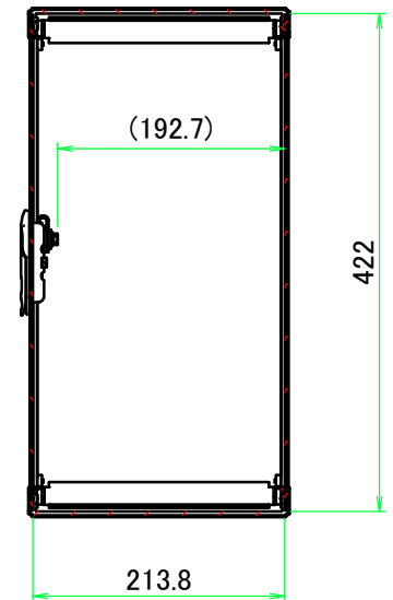
B-B ( 1 : 7 )
