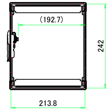
B-B ( 1 : 6.5 )
