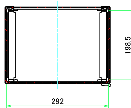
A-A ( 1 : 6.5 )
