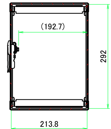
B-B ( 1 : 6.5 )
