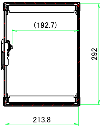
B-B ( 1 : 6.5 )
