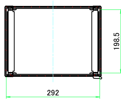
A-A ( 1 : 7 )
