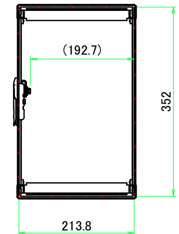
B-B ( 1 : 7 )
