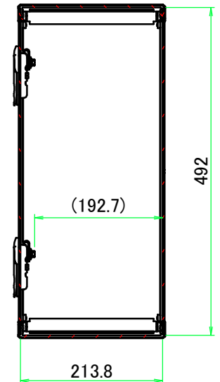
B-B ( 1 : 8 )
