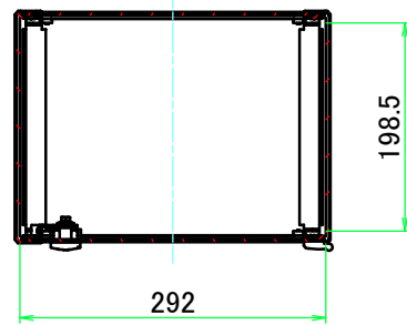
A-A ( 1 : 8 )
