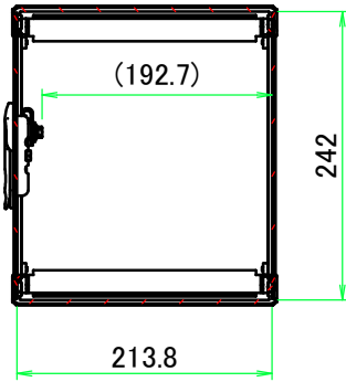
B-B ( 1 : 7 )
