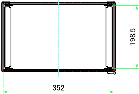
A-A ( 1 : 7 )
