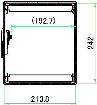
B-B ( 1 : 7 )
