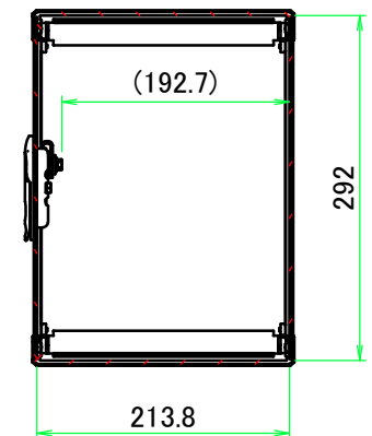
B-B ( 1 : 7 )
