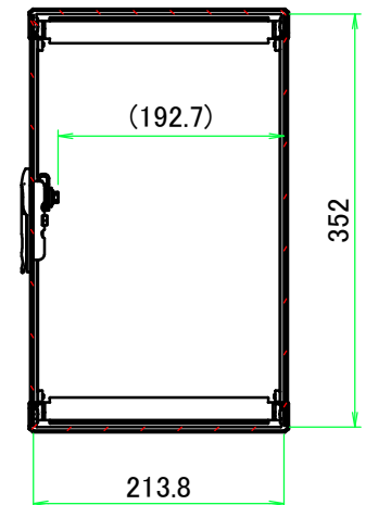
B-B ( 1 : 7 )
