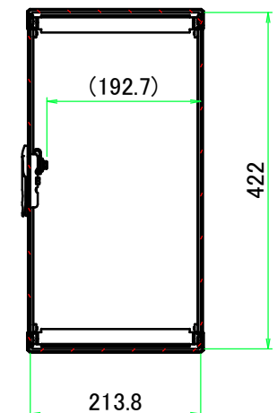
B-B ( 1 : 8.5 )
