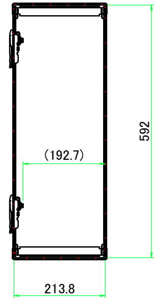
B-B ( 1 : 9 )
