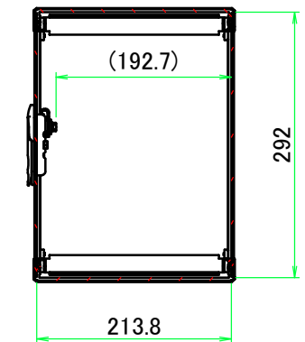
B-B ( 1 : 7.5 )
