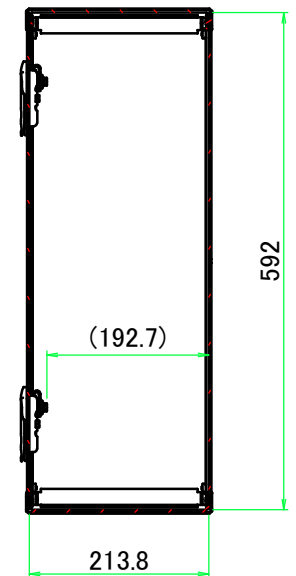
B-B ( 1 : 9 )
