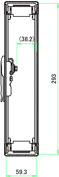
B-B ( 1 : 3.5 )
